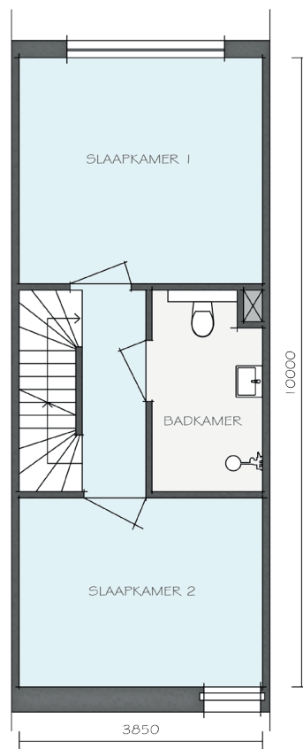
TWEDE VERDIEPING
