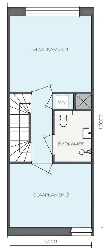
DERDE VERDIEPING
